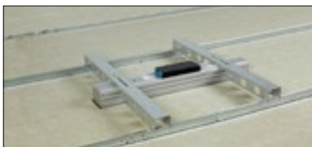
Draagprofielen/paar Voor montage midden in de plafondplaat in verborgen frame, L = 600 mm. Wordt tussen twee profielen gelegd.
